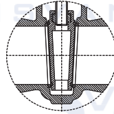
DN125...600 Wedge Type / Sürgü Tipi
